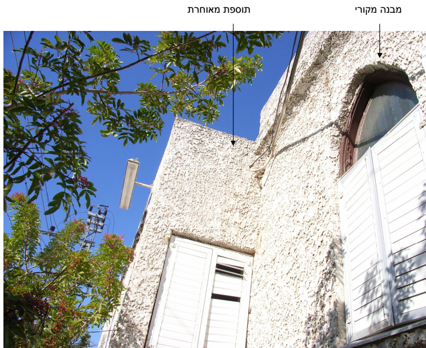
2. חיבור בין התוספת לבין הבית המקורי
